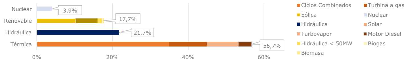
Gráfico 2. Potencia instalada por tipo de tecnología, marzo 2026.
